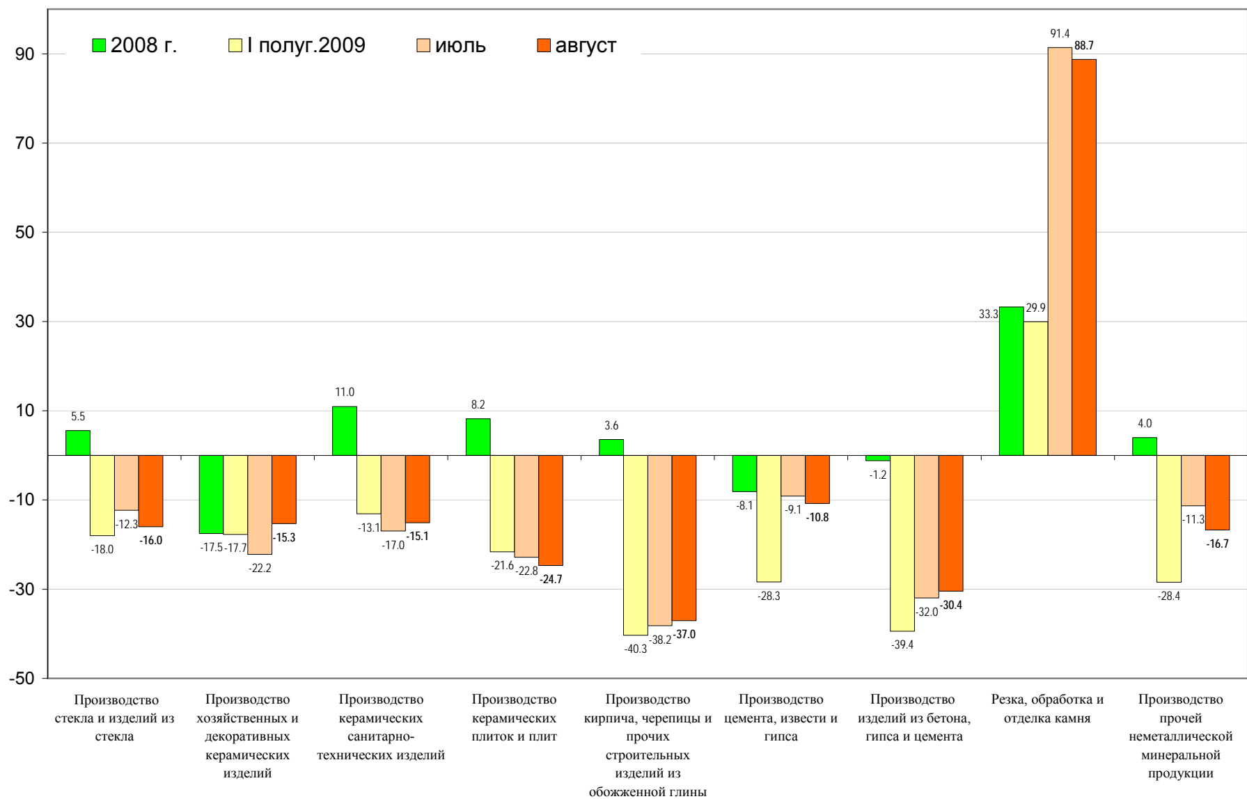
График 8. Динамика производства строительных материалов (темп прироста к соответствующему периоду предшествующего года, %)
